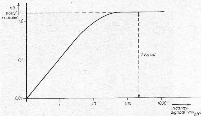
Fig. 5. Conversieversterking van de fasedetector als functie van de amplitude van het ingangssignaal.
