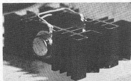
Afb. 5. Gestabiliseerde voeding met LM 309K.
