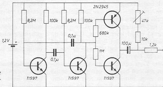
Fig. 1. Schakeling van de elektronische botgroeistimulator.
