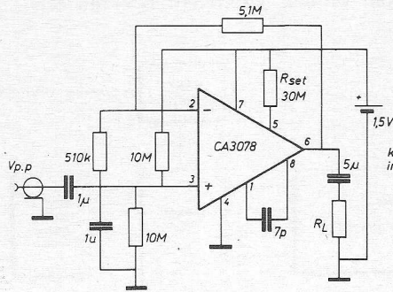
Fig. 7. Niet-inverterende versterker.
