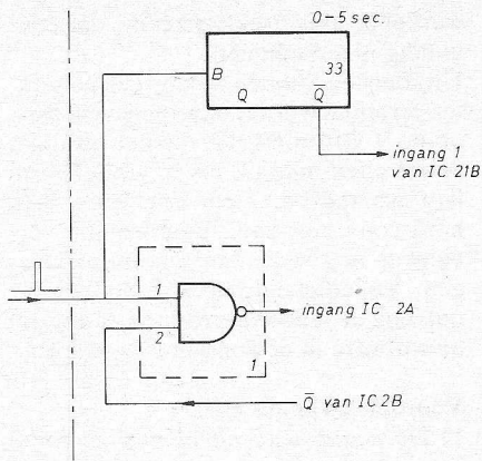
Fig. 22. Patiëntbewaking.
