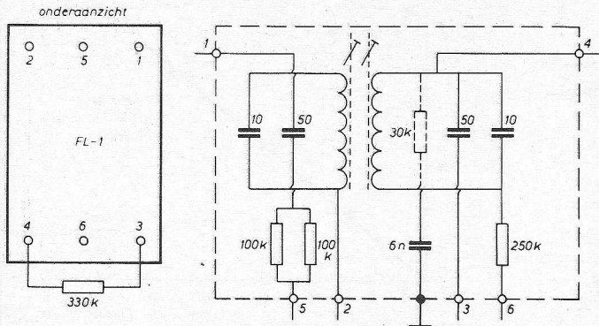
Fig. 7. De inhoud van spoelbus FL 1 met zijn aansluitpunten. De weerstand van 30 kΩ is verwijderd. Uitwendig wordt 330 kΩ gemonteerd tussen de punten 3 en 4.
