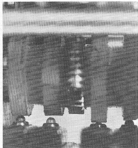
Afb. 2. Detail van het roermechanisme. Duidelijk zijn de nokken en microscharakelaar zichtbaar.
