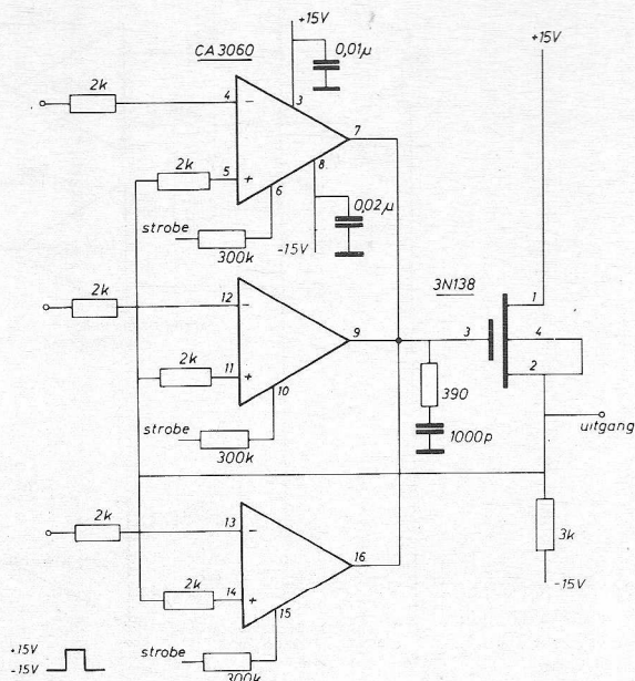
Fig. 4. Multiplexer met drie kanalen.
