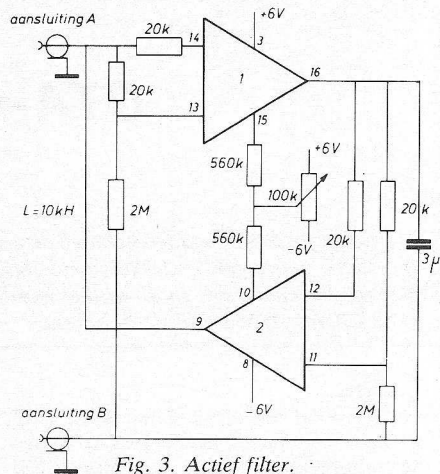
Fig. 3. Actief filter.
