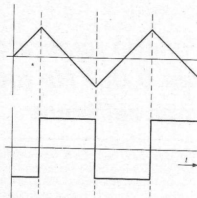
Fig. 2. Uitgangsspanning van integrator resp. discriminator.
