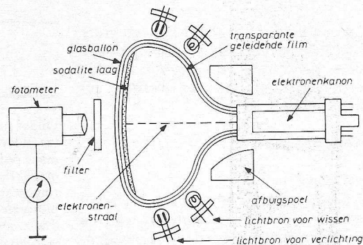
Fig. 1. Fundamentele doorsnede van een kathodochrome buis en het contrast-meetsysteem.
