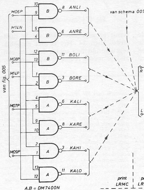
Fig. 7. Decodeerschakeling van de motorcommando's.
