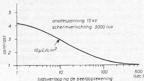
Fig. 3. Nabeeldtijd karakteristieken.
