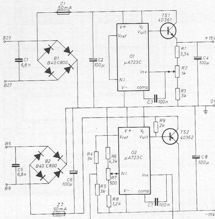
Fig. 18. De dubbele voeding, 2 x 15 V, is op print B gesitueerd.
