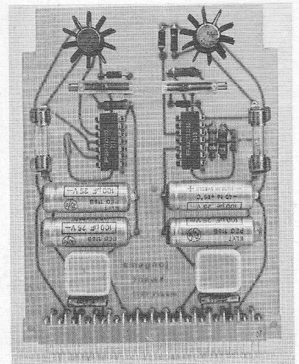
Fig. 18. De dubbele voeding, 2 x 15 V, is op print B gesitueerd.
