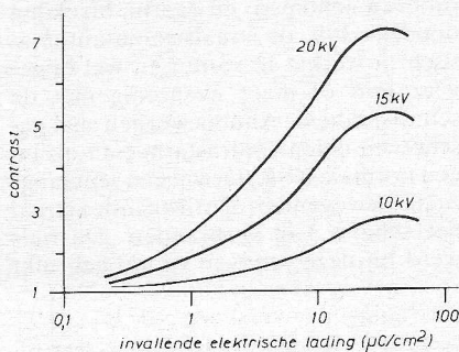
Fig. 2. Contrastkarakteristieken van sodalite.
