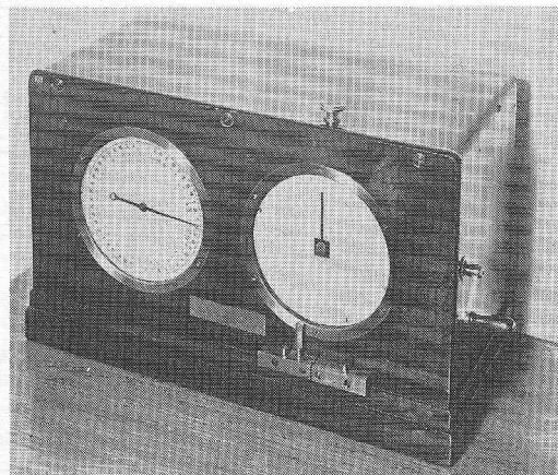
Wijzertelegraaf van E. Wenckebach. Links de schaal met alfabet en cijfers, rechts een galvanometer voor controle van de lijnstroom (1845). Aan de rechterzijde de kruk voor het bedienen van het impulscontact.
