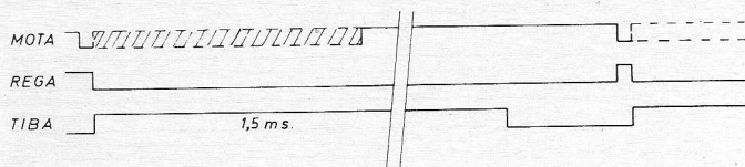
Tijddiagram 2: starten van de tijdbasis.
