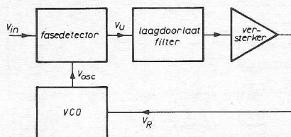
Fig. 1. Blokschema van een fasevergelingschakeling.
