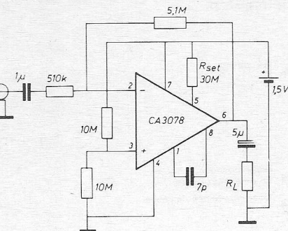
Fig. 6. Inverterende versterker.
