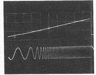
Afb. 4. „Gesweepte” VCO. Realisatie: 1) Sweep driehoek asymm. 2) VCO hiermee gesweept.
