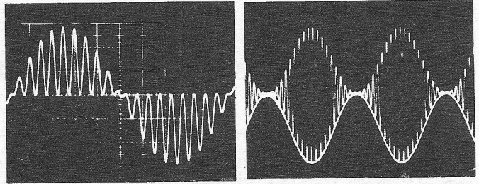
Fig. 5. Golfvormen van de twee kwadranten vermenigvuldiger.
