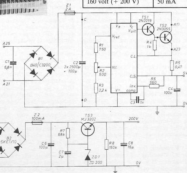
Fig. 19. Voedingen voor resp. 5 V en 200 V, ondergebracht op een gemeenschappelijk printje.
