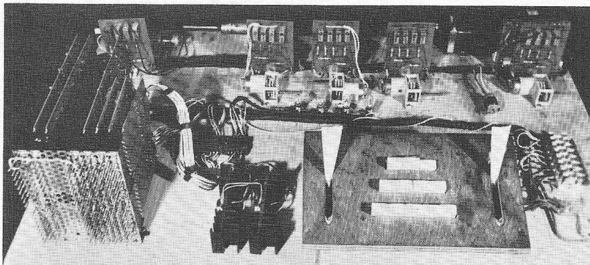
Afb. 6. Totaaloverzicht van de experimentele schakeling. Links de zender/ontvanger, op de achtergrond de motoren en de lampjes (met stureenheden), op de voorgrond de gecombineerde voeding en het bedieningspaneel.
