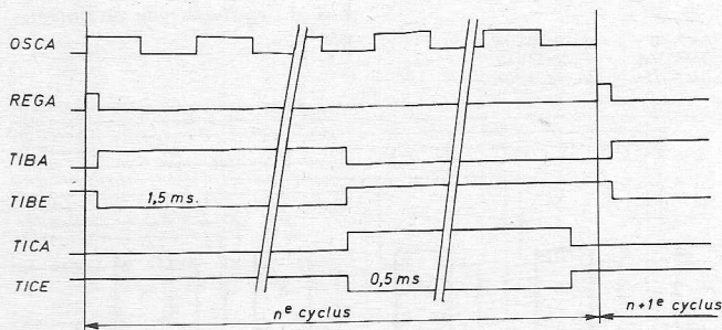
Tijddiagram 1: tijdbasis.
