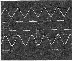
Afb. 1. Uitgangsignalen van sweep en VCO.
