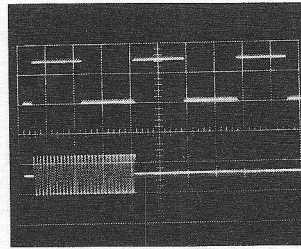
Afb. 3. Burst-opwekking. Realisatie: SK 1202 op 1 cyclus, daarna drukken op SK 1201 of ext. signaal.
