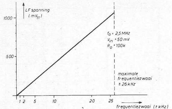
Fig. 6. Het verband tussen LF-gemoduleerd signaal en de frequentiezwaai voor een XR 210.
