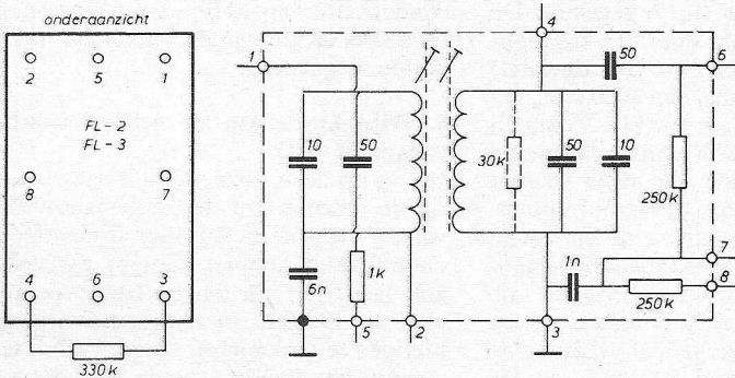
Fig. 8. De inhoud van spoelbus FL 2 en FL 3 met zijn aansluitgegevens. Ook hierbij worden dezelfde handelingen verricht als bij fig. 7.
